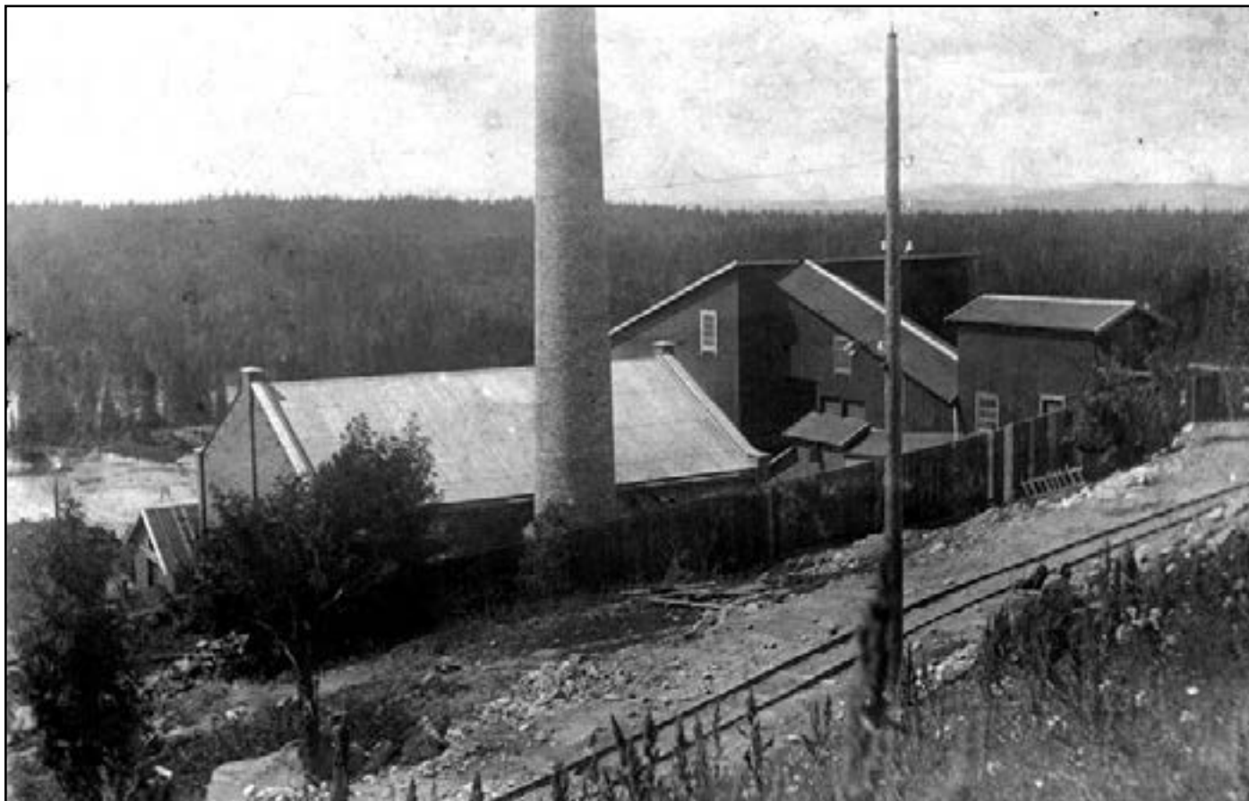
Fabrikken sett fra sør-øst. I forgrunnen sees jernbanen der malmen ble fraktet fra gruva til pukkverket. Den pukkede malmen ble heist inn i verket gjennom den skråstilte bygningen. Bygningen bak fabrikkpipa er maskinhuset. En lysstolpe sees helt i forgrunnen. (Foto utlånt av Oleif Hoel, Eidsvoll)
