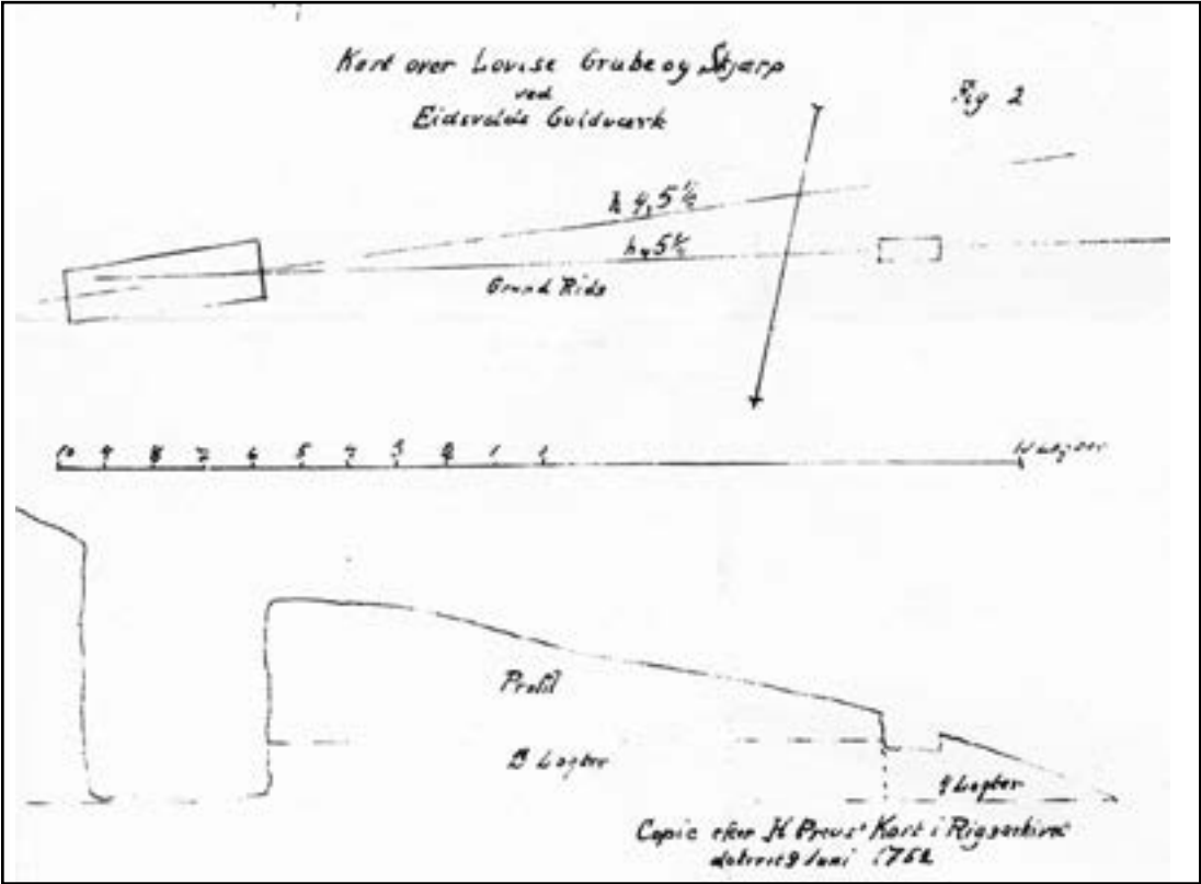
Snitt av Prinsesse Louises gruve. Kartet sies å være en kopi av H. Preus' kart i Riksarkivet, datert 9. juni 1752, altså fra kobberverkets tid. (Fra NTHs opptrykk av D. E. Bradts bok om gullverket fra 1790)
