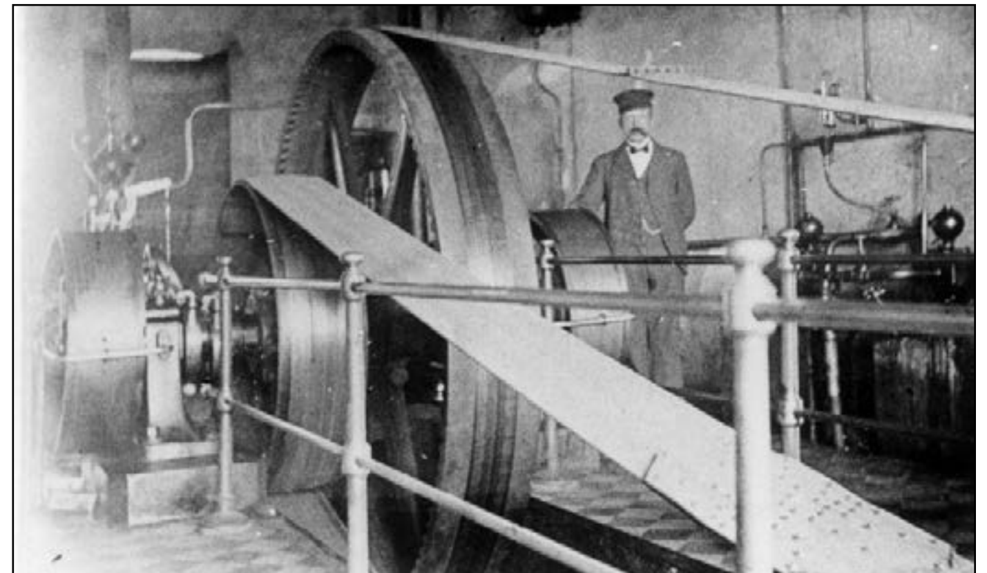
Interiørbilde fra maskinhuset. Legg merke til det flislagte golvet og dimensjonen på svinghjulet. Mannen på bildet er maskinist Hans Hagen. (Foto utlånt av Oleif Hoel, Eidsvoll).
