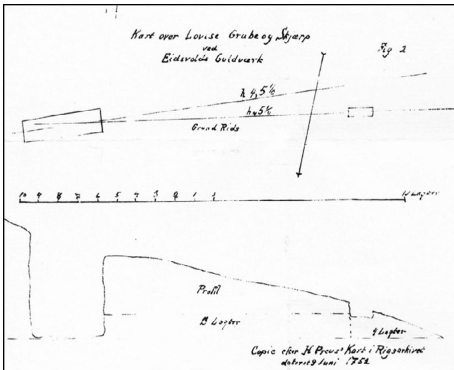
Snitt av Prinsesse Louises gruve. Kartet sies å være en kopi av H. Preus' kart i Riksarkivet, datert 9. juni 1752, altså fra kobberverkets tid. (Fra NTHs opptrykk av D. E. Bradts bok om gullverket fra 1790)
