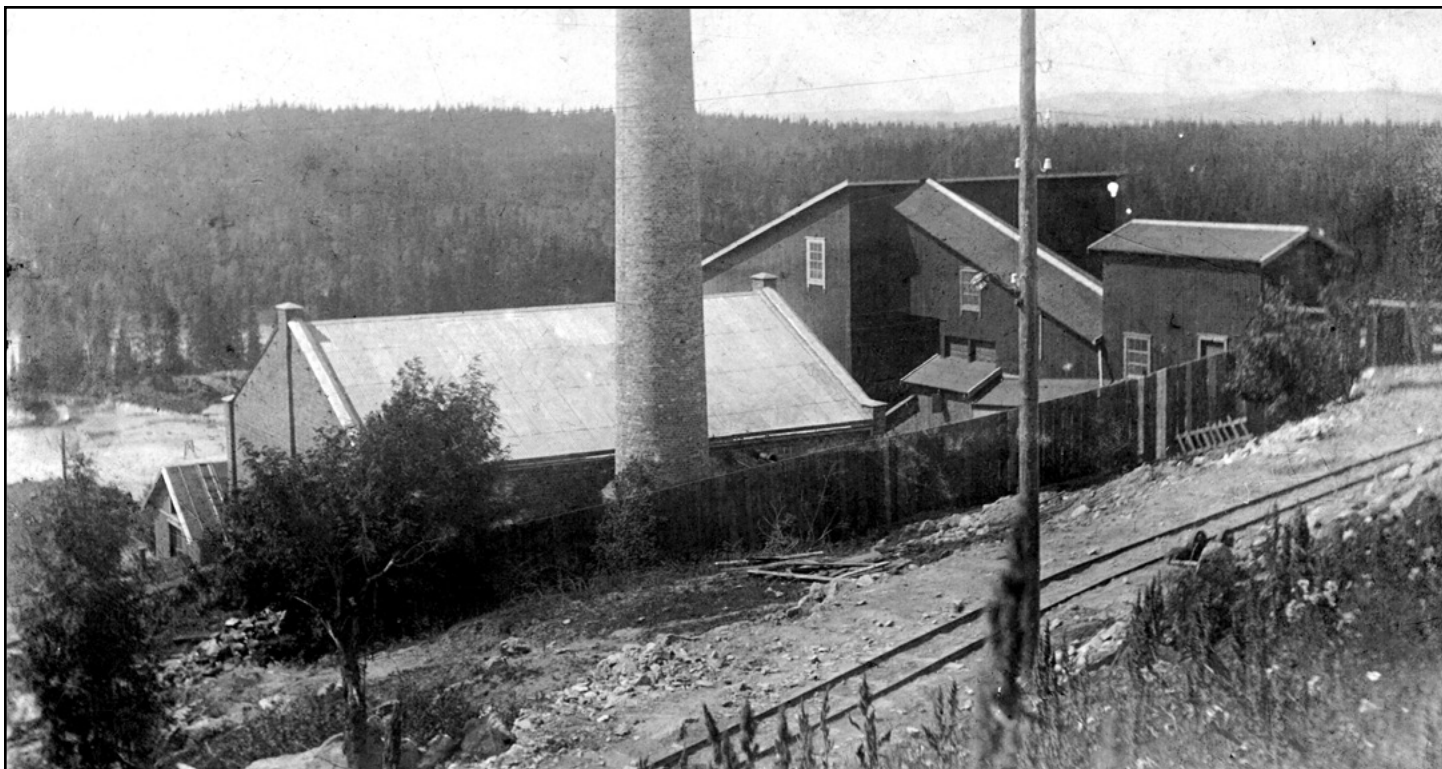
Fabrikken sett fra sør-øst. I forgrunnen sees jernbanen der malmen ble fraktet fra gruva til pukkverket. Den pukkede malmen ble heist inn i verket gjennom den skrånede bygningen. Bygningen bak fabrikkpipa er maskinhuset. En lysstolpe sees helt i forgrunnen. (Foto utlånt av Oleif Hoel, Eidsvoll)
